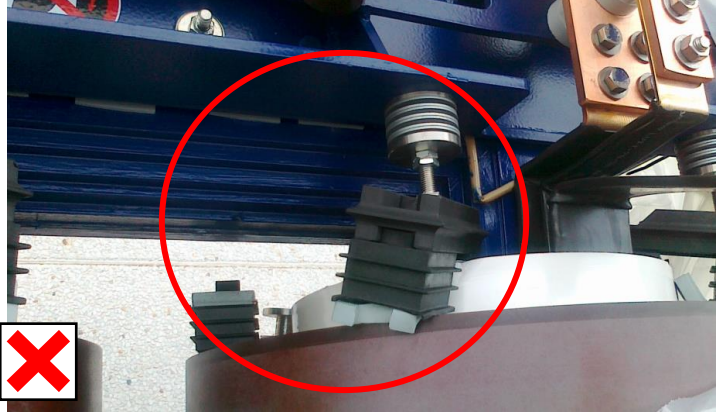
Şek. 15: Yasak! Sarımlar kaydırmış. Devrilmiş desteklerden anlaşılır.
