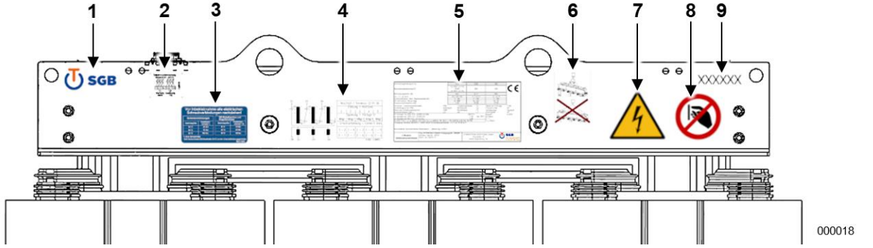
Şek. 26: Üst presleme demirinin OS tarafındaki yazı (Örnek)
