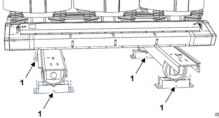
Şek. 19: Transformatör yatağı
